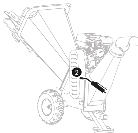
Schmierstellen Trommelhackwerk
