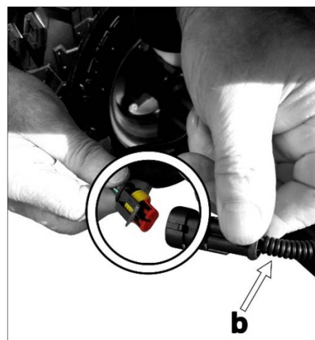
Sicherheitsschaltung (NOT-HALT) anschließen
