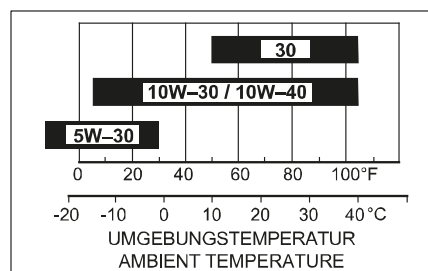
Motoröl Viskosität
