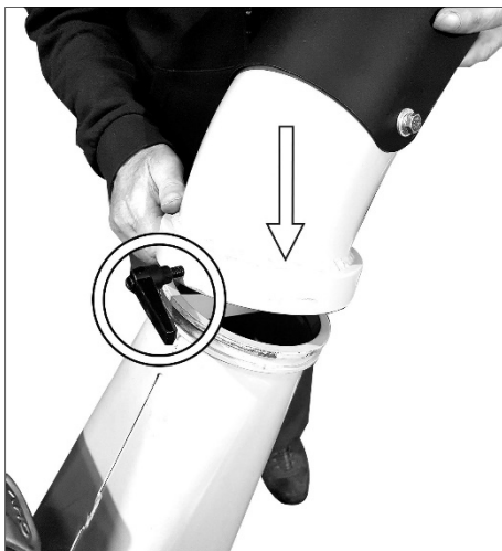
Auswurfklappe montieren
